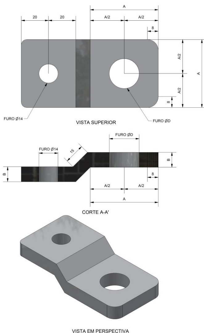
Figura 1 - Chapa Curva para Aterramento de Cadeia de Isoladores
